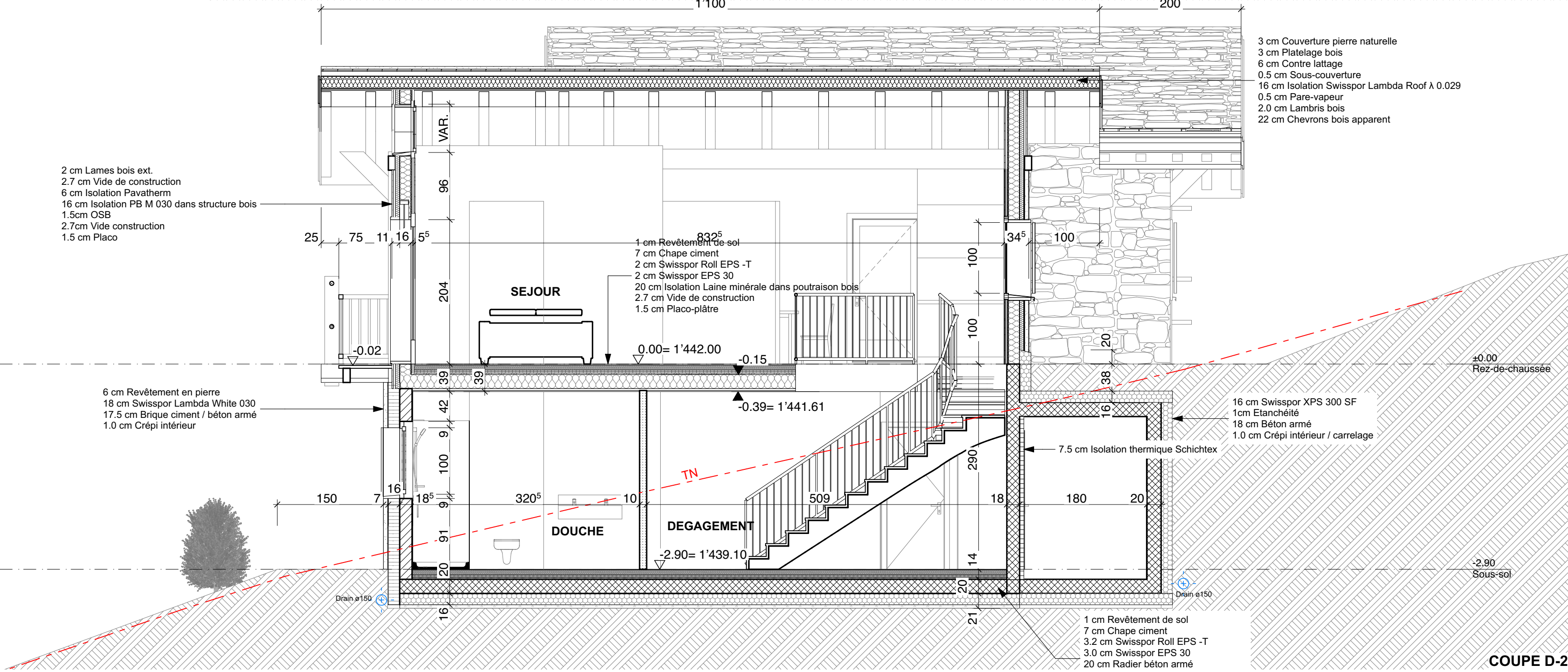
COUPE D-2
