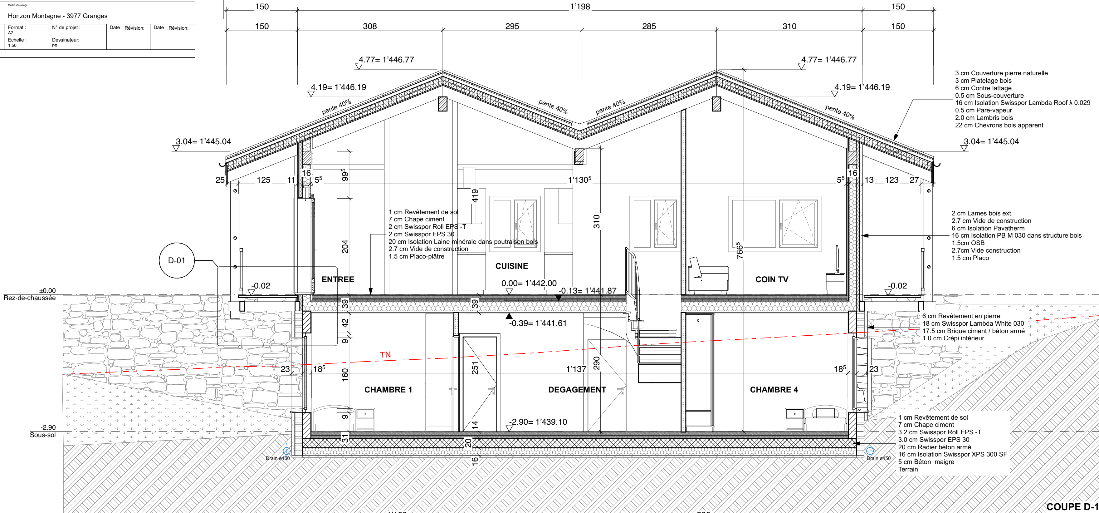
COUPE D-1
